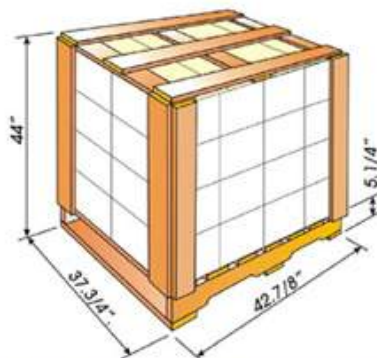
SA pallet Type A (44 Cartons)
