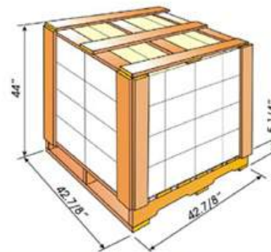
SA pallet Type B (48 Cartons)
